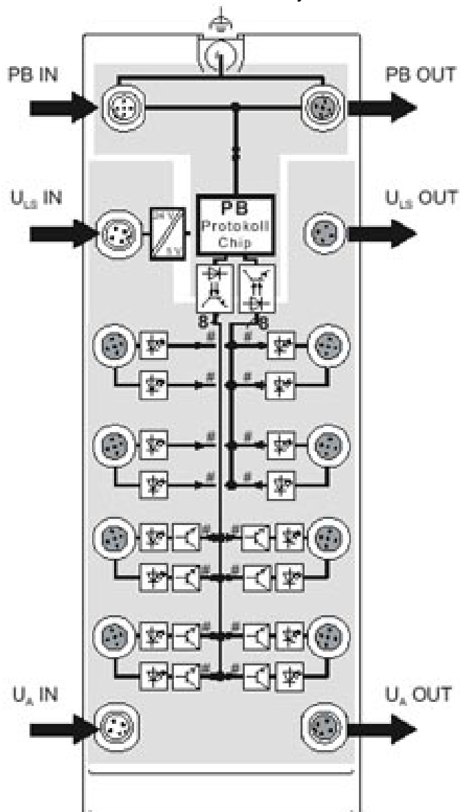
Schemat blokowy
