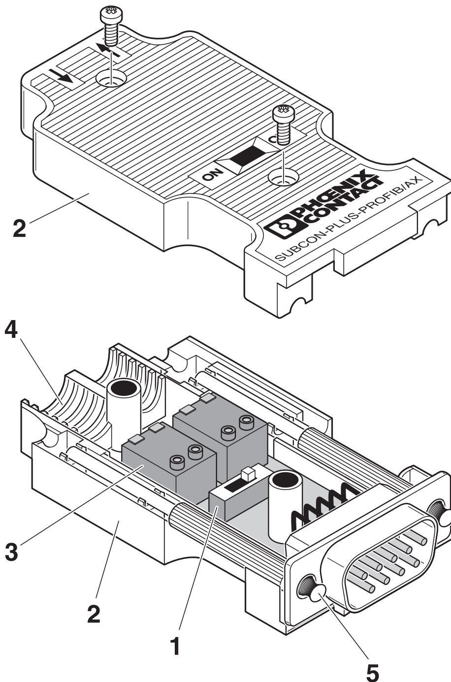
Rysunek schematyczny
