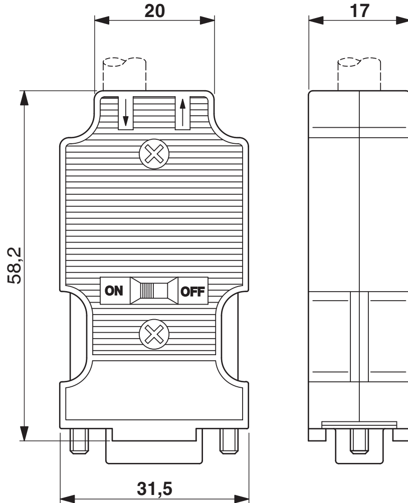
Rysunek wymiarowy
