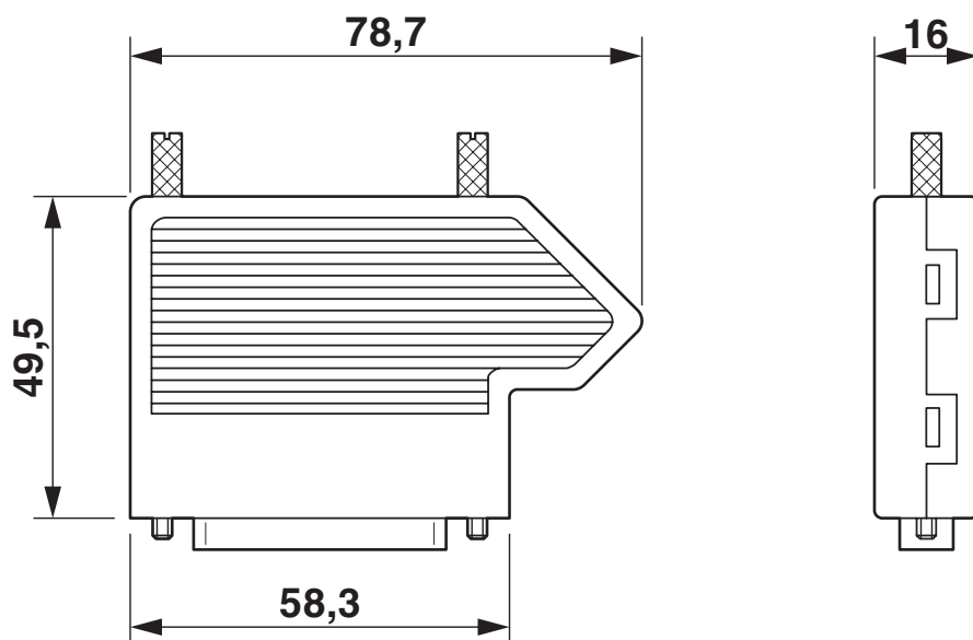
Rysunek wymiarowy
