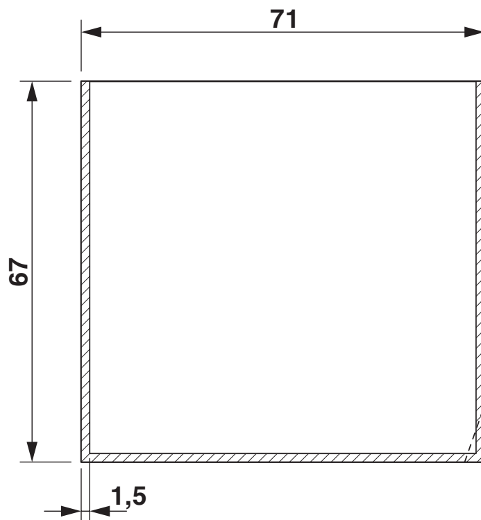
Rysunek wymiarowy
