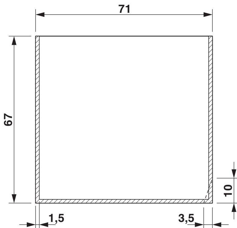
Rysunek wymiarowy
