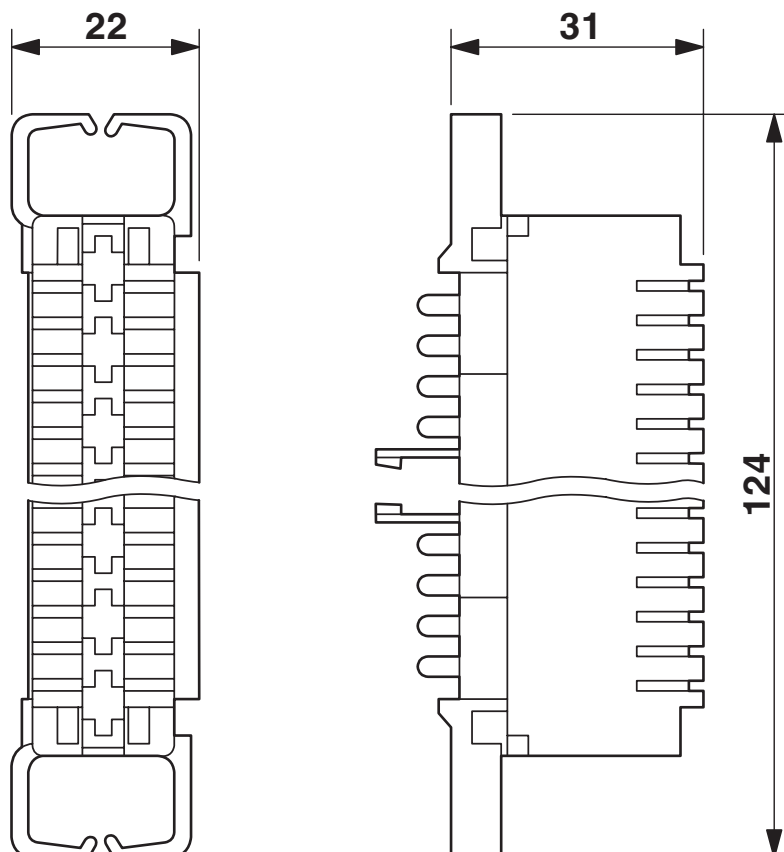
Rysunek wymiarowy
