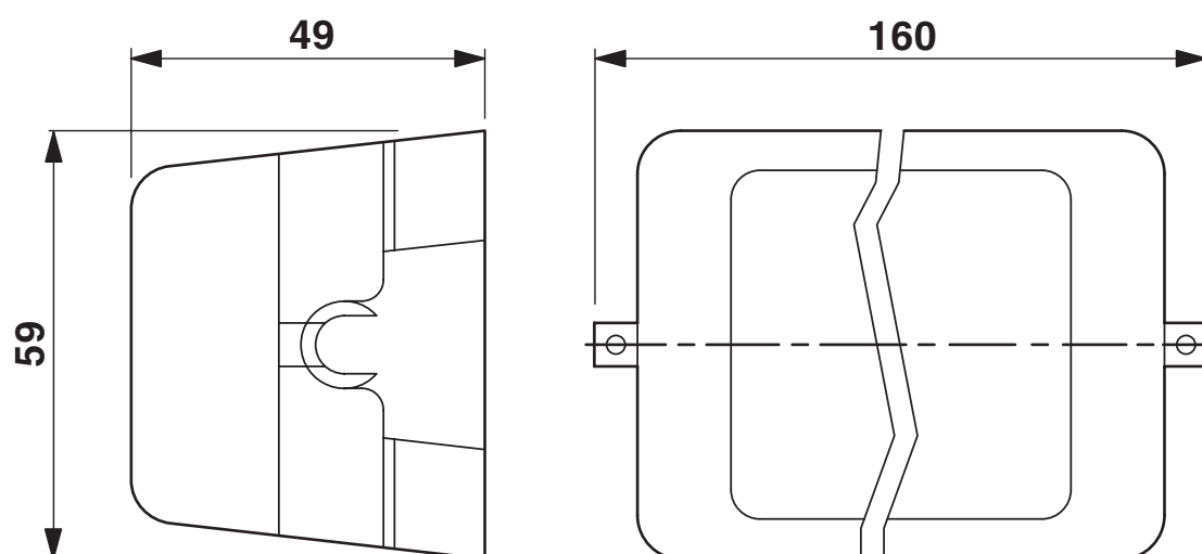
Rysunek wymiarowy
