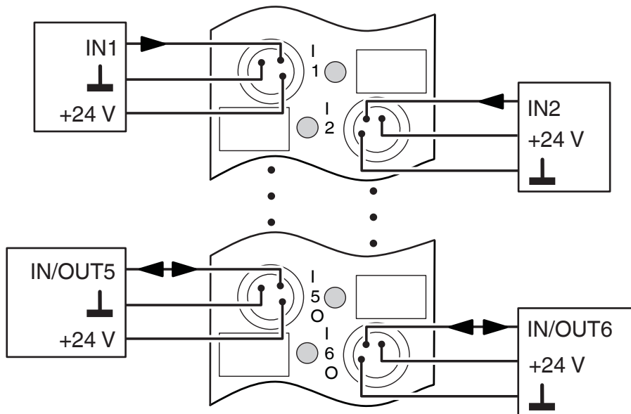
rysunek złączy
