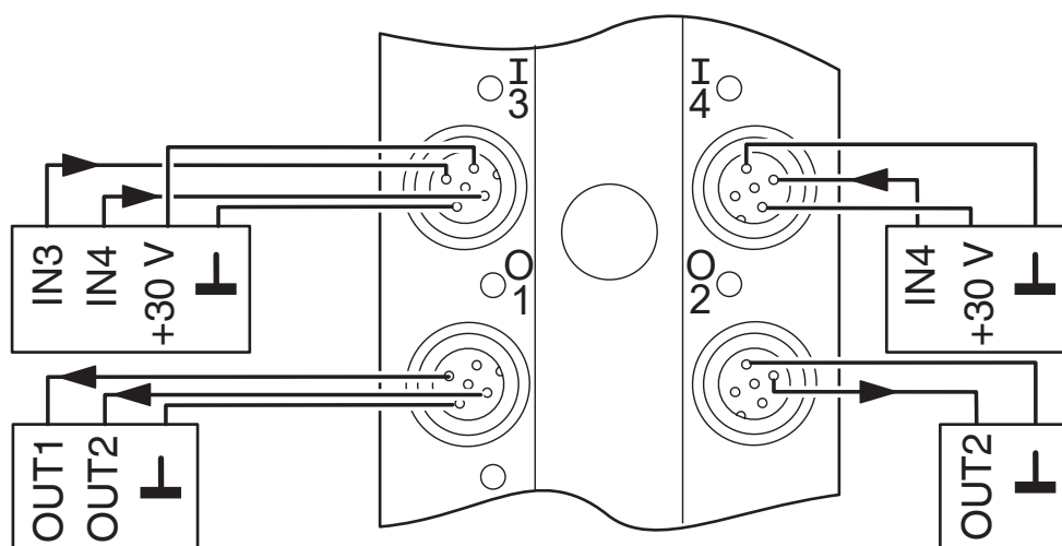
rysunek złączy
