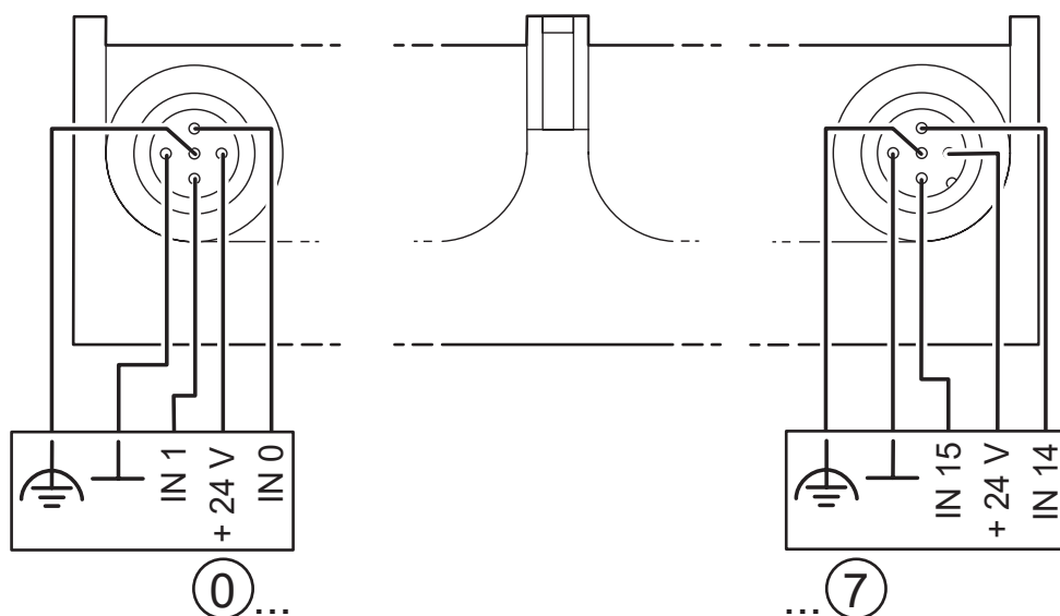
rysunek złączy
