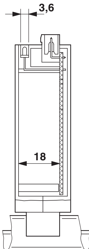
Rysunek wymiarowy
