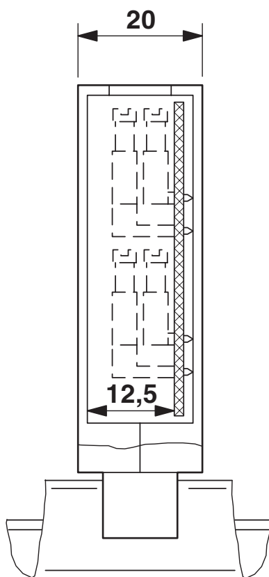
Rysunek wymiarowy
