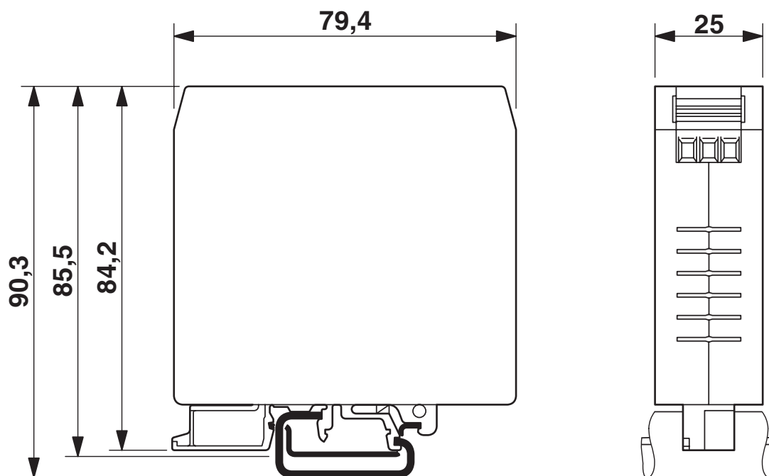
Rysunek wymiarowy
