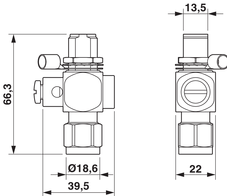
Rysunek wymiarowy
