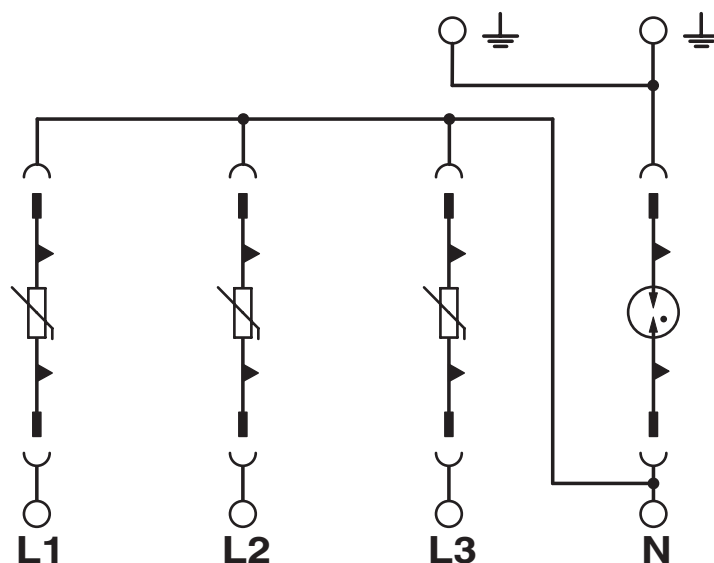
Schemat
