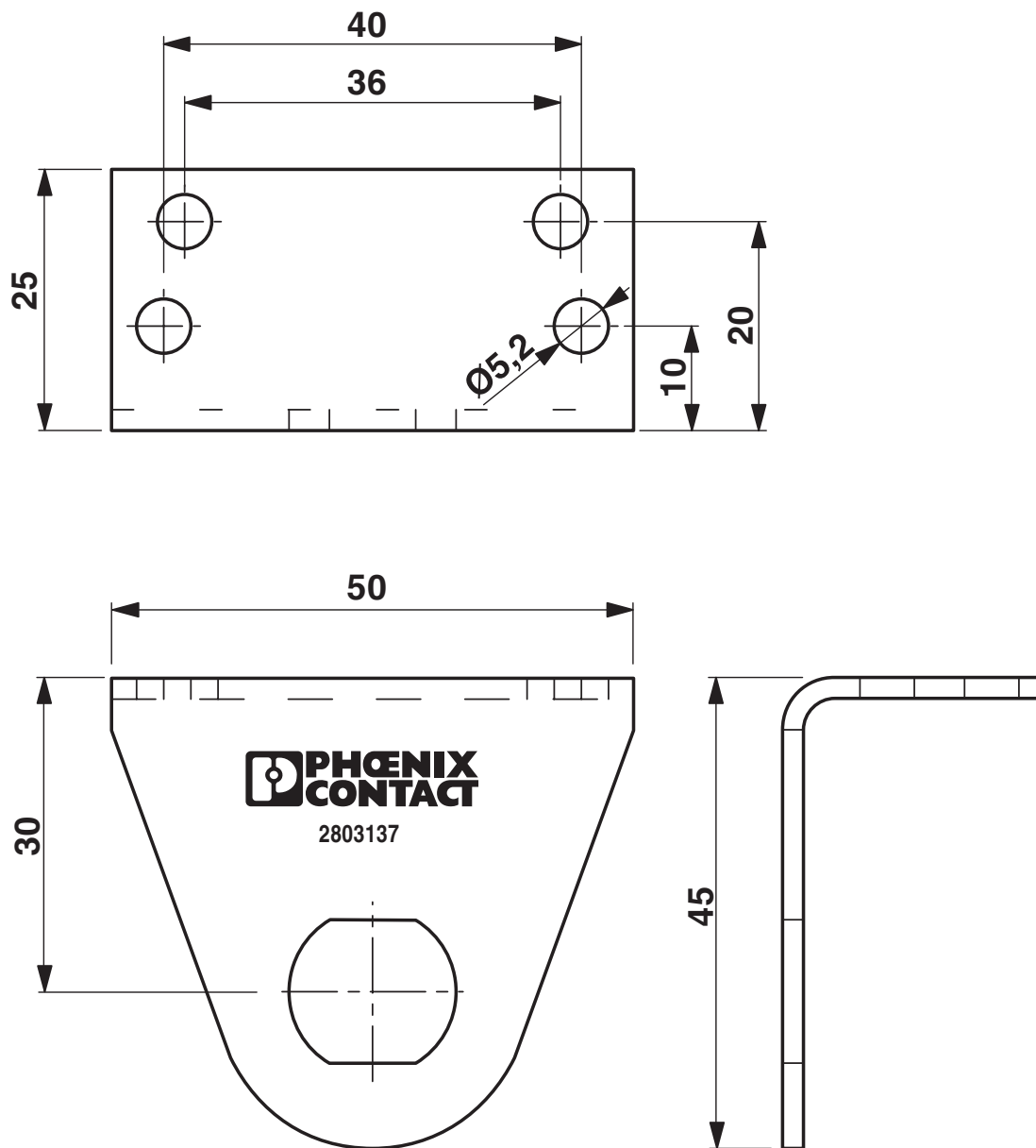
Rysunek wymiarowy
