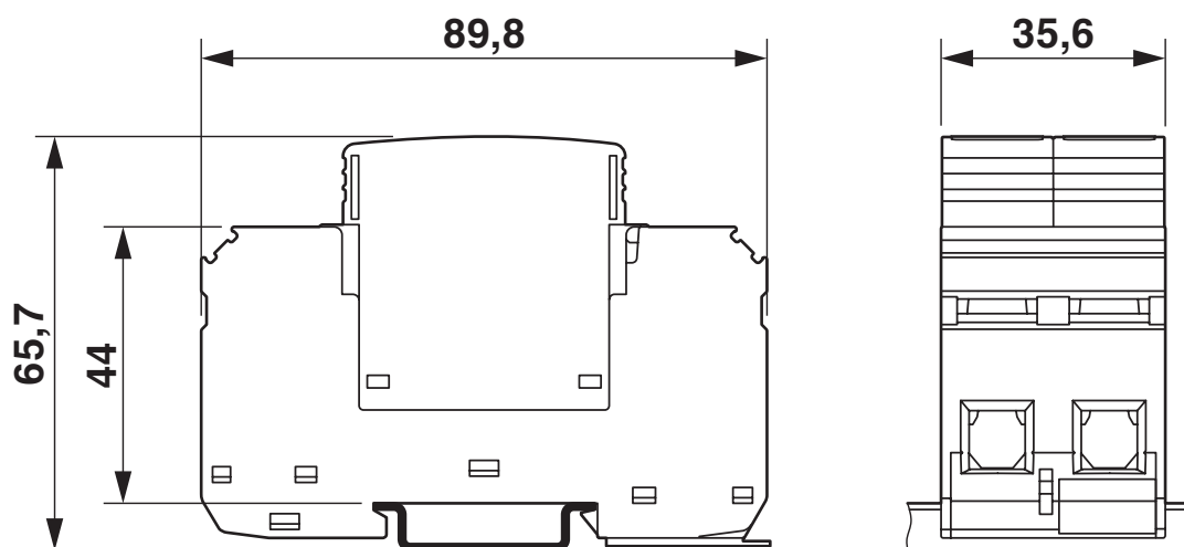
Rysunek wymiarowy
