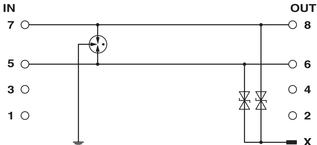
Schemat
