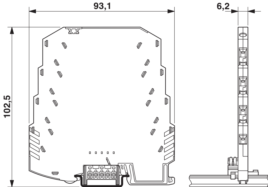
Rysunek wymiarowy
