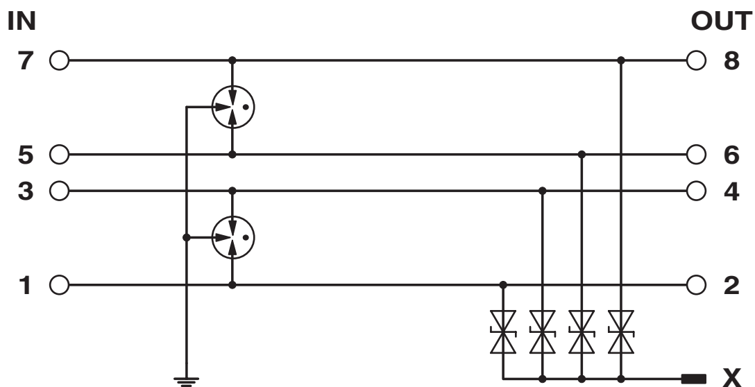
Schemat
