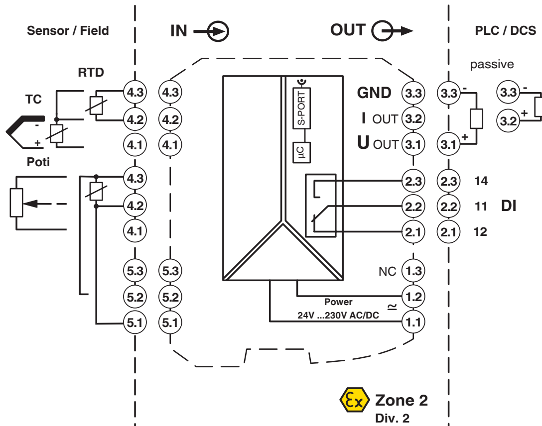
Schemat blokowy
