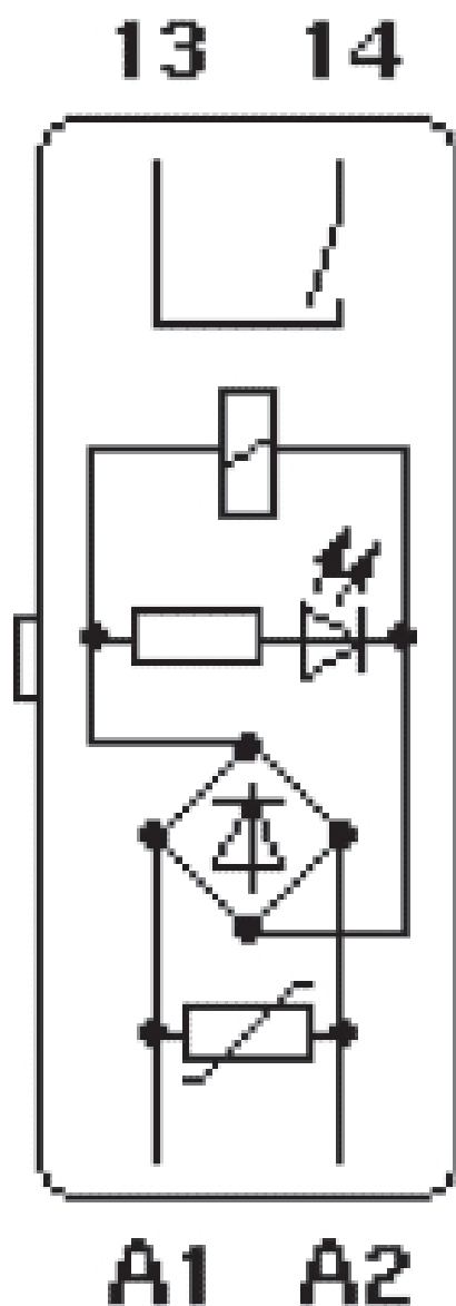
Schemat
