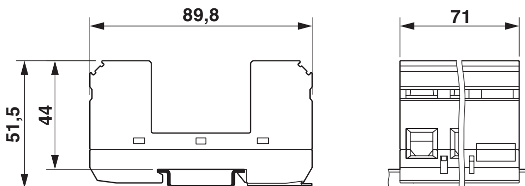
Rysunek wymiarowy
