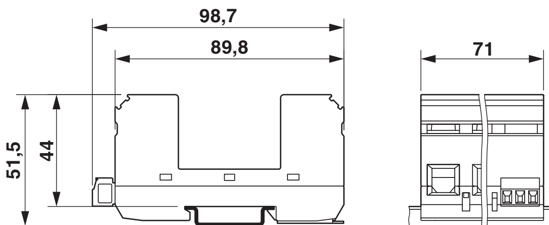
Rysunek wymiarowy
