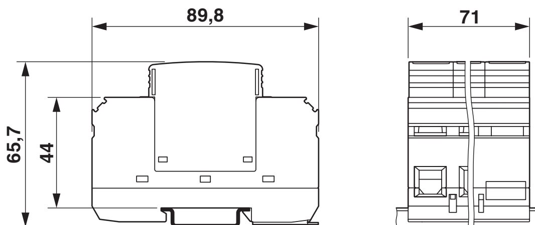
Rysunek wymiarowy
