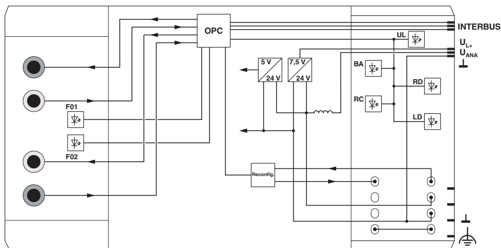
Schemat blokowy
