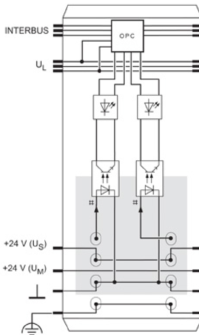
Schemat blokowy
