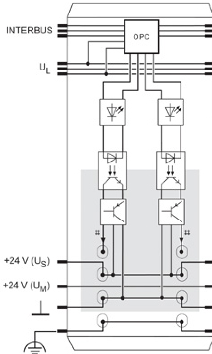
Schemat blokowy
