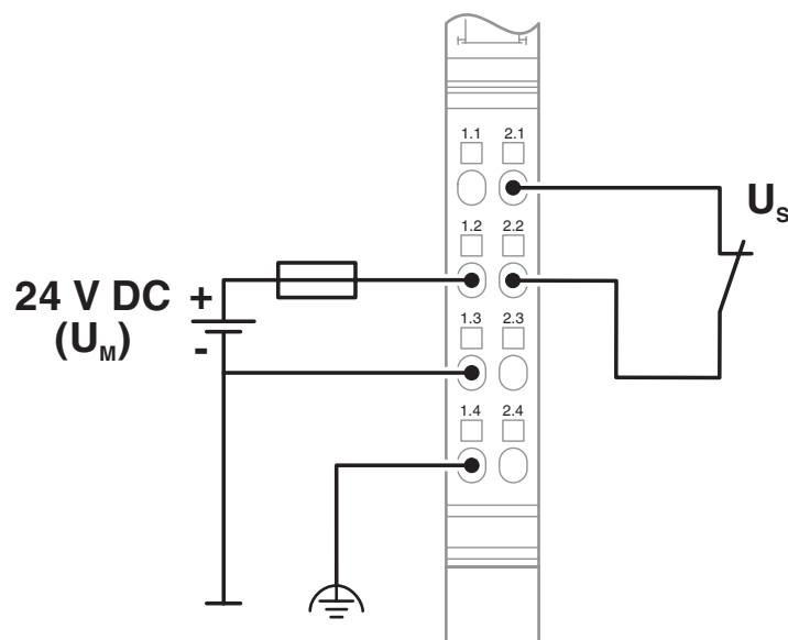
rysunek złączy
