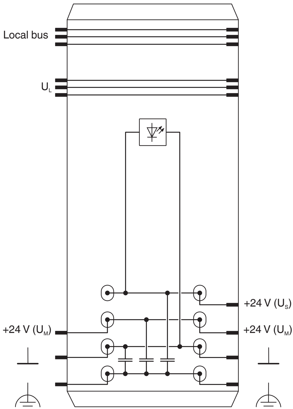
Schemat blokowy
