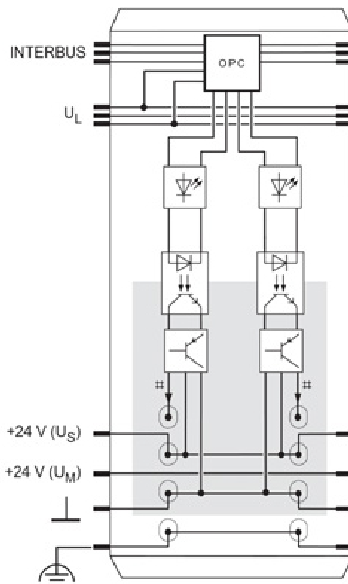
Schemat blokowy
