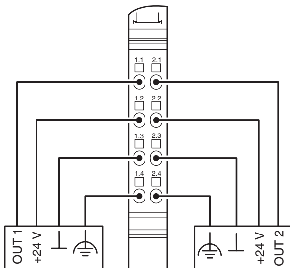
rysunek złączy
