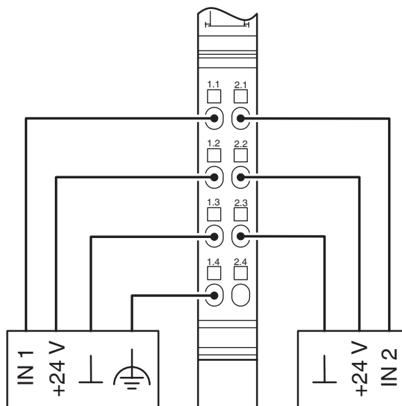
rysunek złączy
