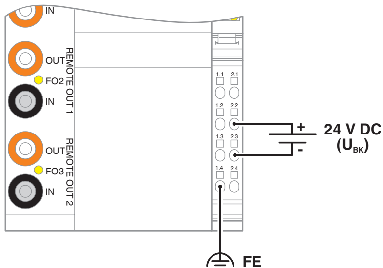
rysunek złączy
