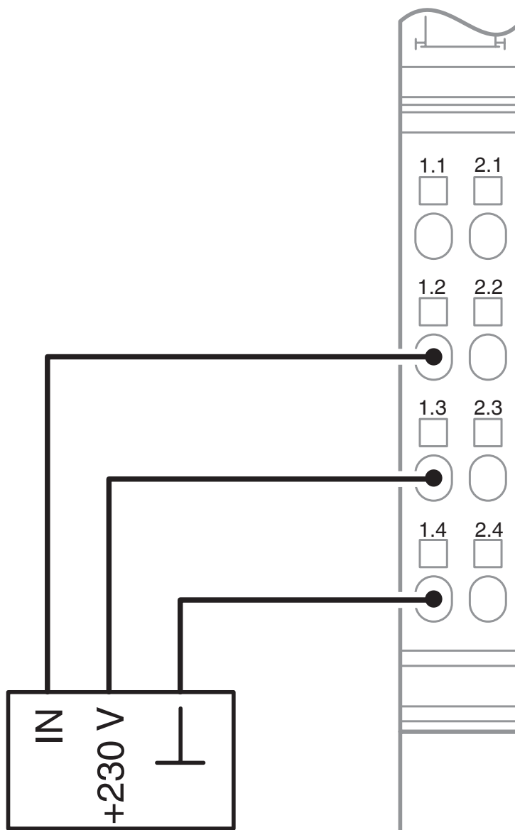
rysunek złączy
