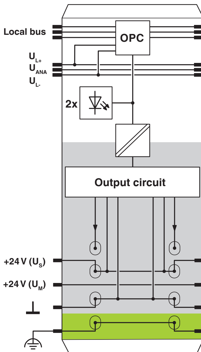
Schemat blokowy
