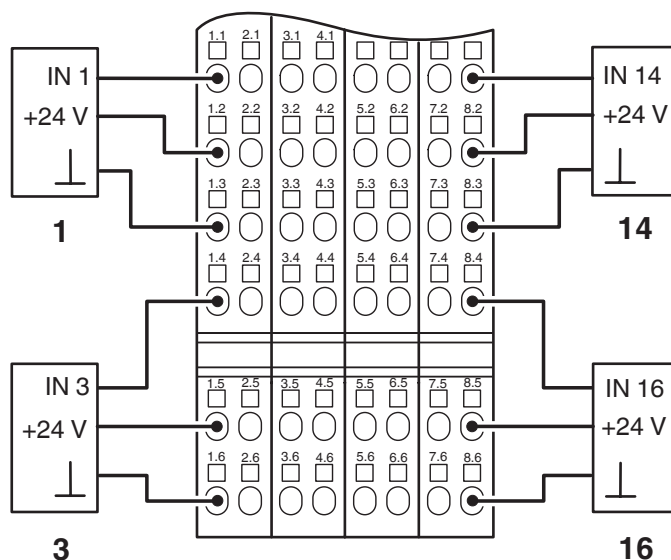
rysunek złączy
