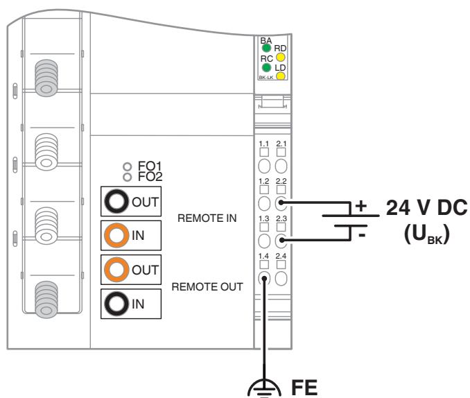
rysunek złączy
