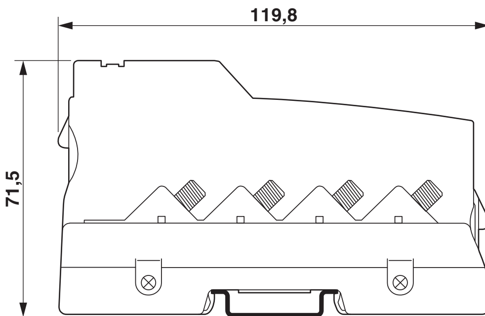
Rysunek wymiarowy
