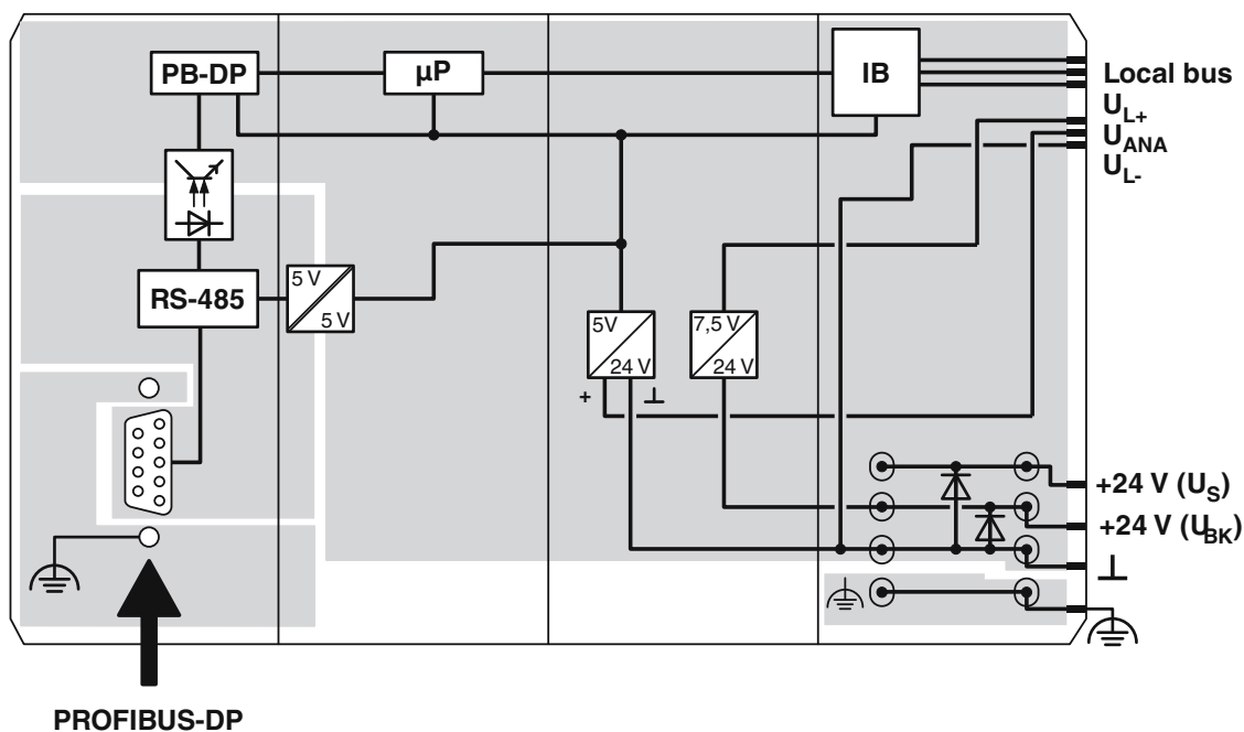
Schemat blokowy
