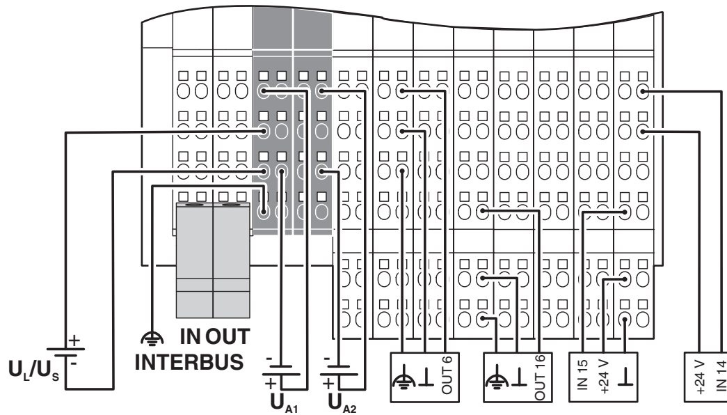
rysunek złączy
