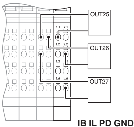
rysunek złączy
