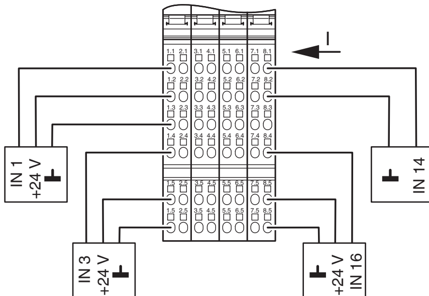
rysunek złączy
