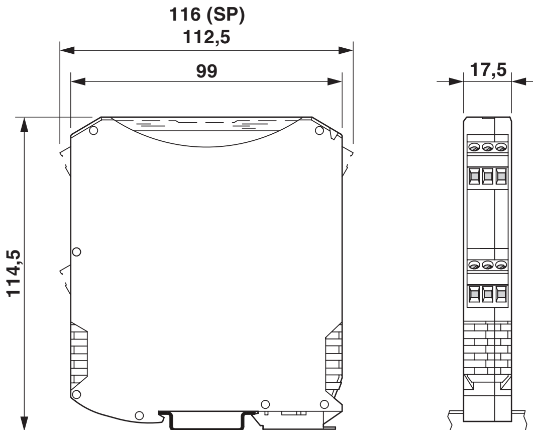
Rysunek wymiarowy
