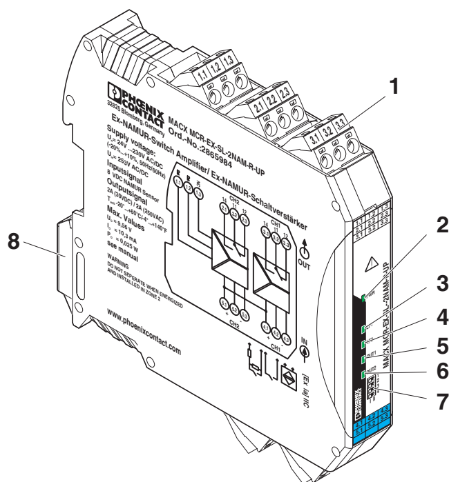
Rysunek schematyczny
