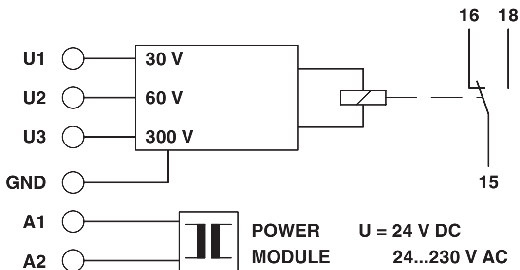
Schemat blokowy
