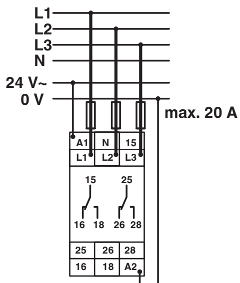
rysunek aplikacji
