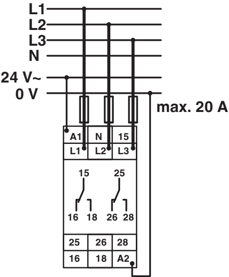
rysunek złączy
