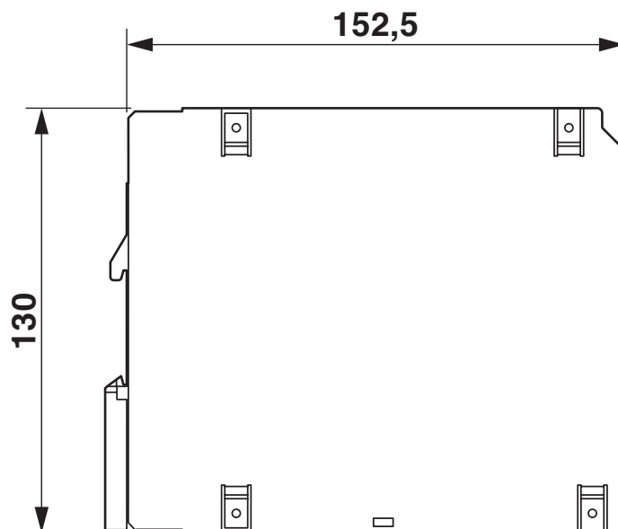
Rysunek wymiarowy
