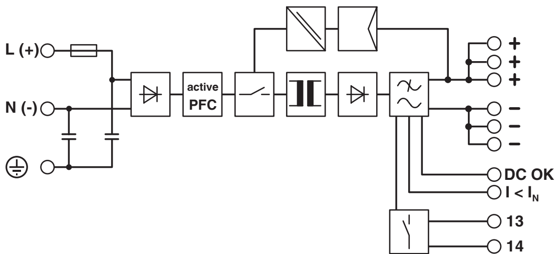
Schemat blokowy
