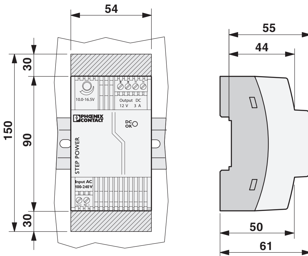
Rysunek wymiarowy
