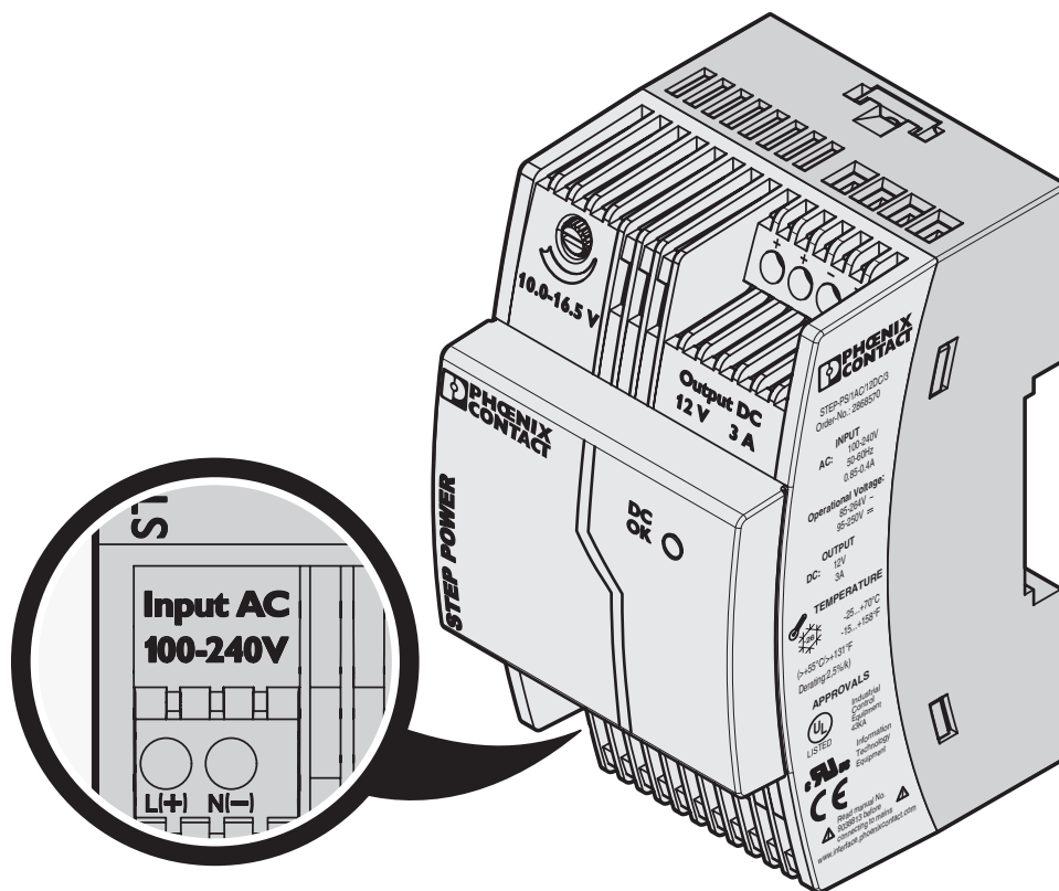
Rysunek schematyczny
