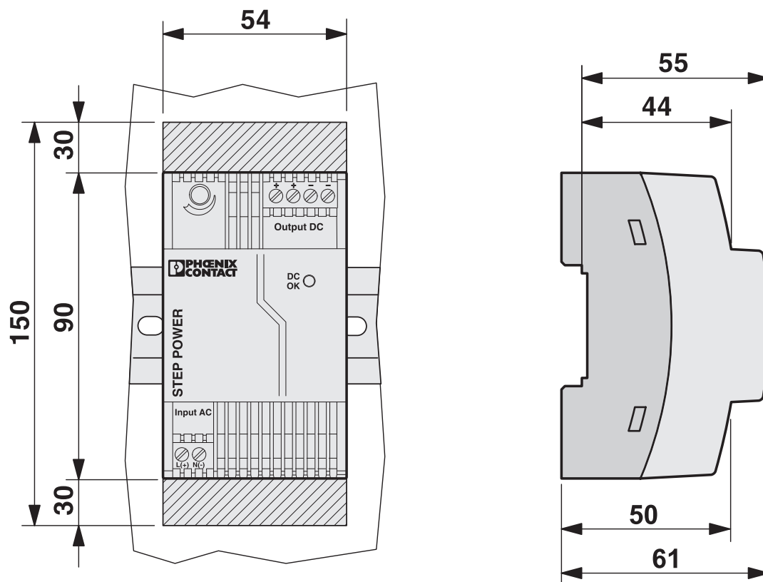
Rysunek wymiarowy
