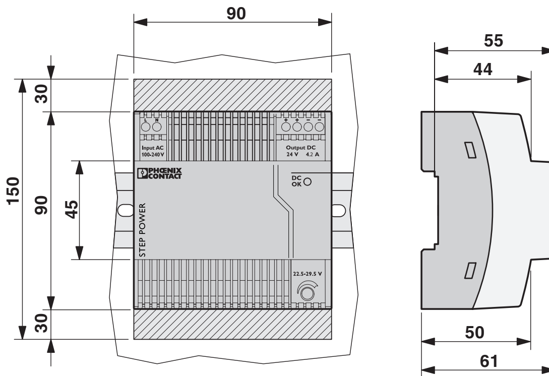
Rysunek wymiarowy
