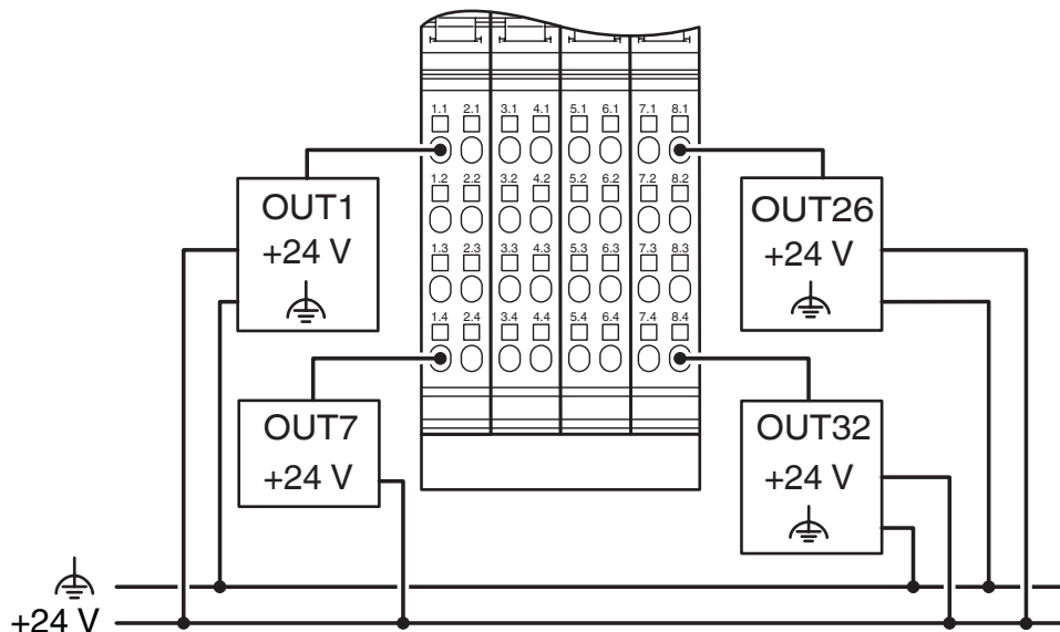
rysunek złączy
