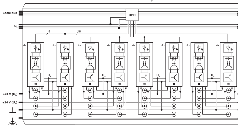
Schemat blokowy
