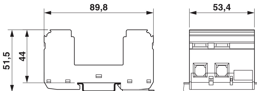
Rysunek wymiarowy
